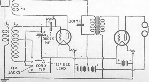
Circuito de ondas corta.—(Véase la descripción.)
